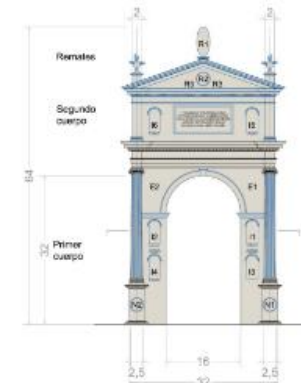
Alzado principal u occidental, a las cuatro calles
